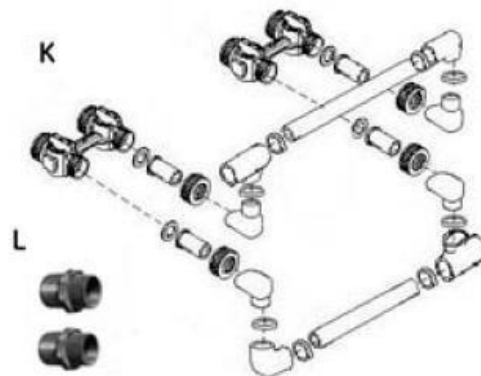
Рис 12 – 278-764 - монтажный для комплект для параллельной системы
