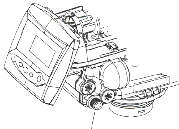
Место подключения реактентной трубки
