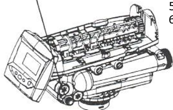
Ограничитель потока заполнения реagenтного бака
