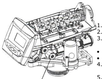
Эжектор и крышка
